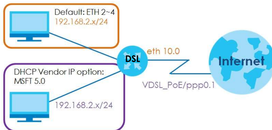
Obrázek 76 Příklad slučování rozhraní
