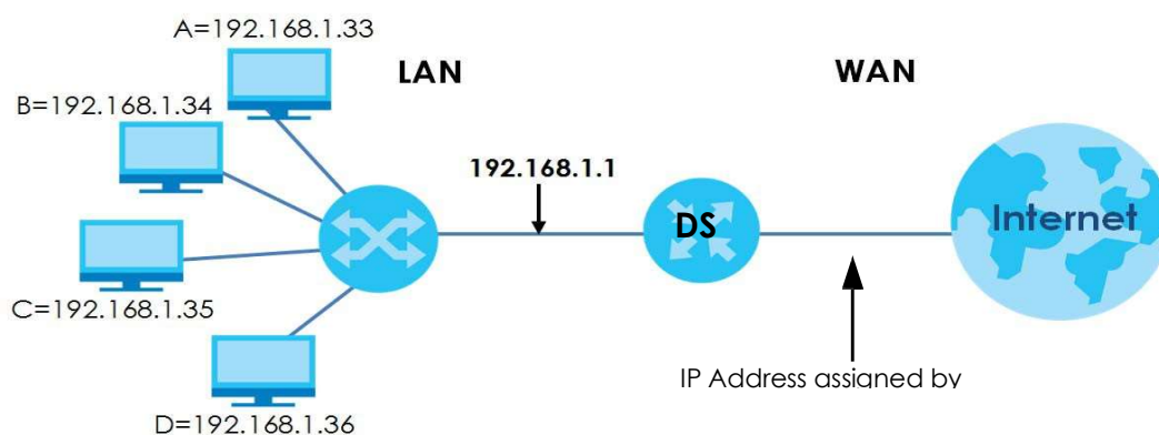
Obrázek 60 Více serverů za NATem (příklad)
